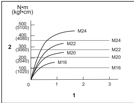
1. Masa pengikat (saat) 2. Tork pengikat
