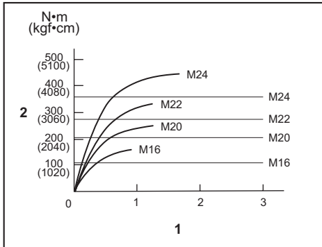
1. Thời gian vận xiết (giây) 2. Lực vận xiết
