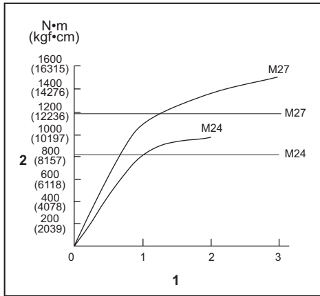
1. เวลาการขันแน่น (วินาที) 2. แรงบิดขั้นแน่น
